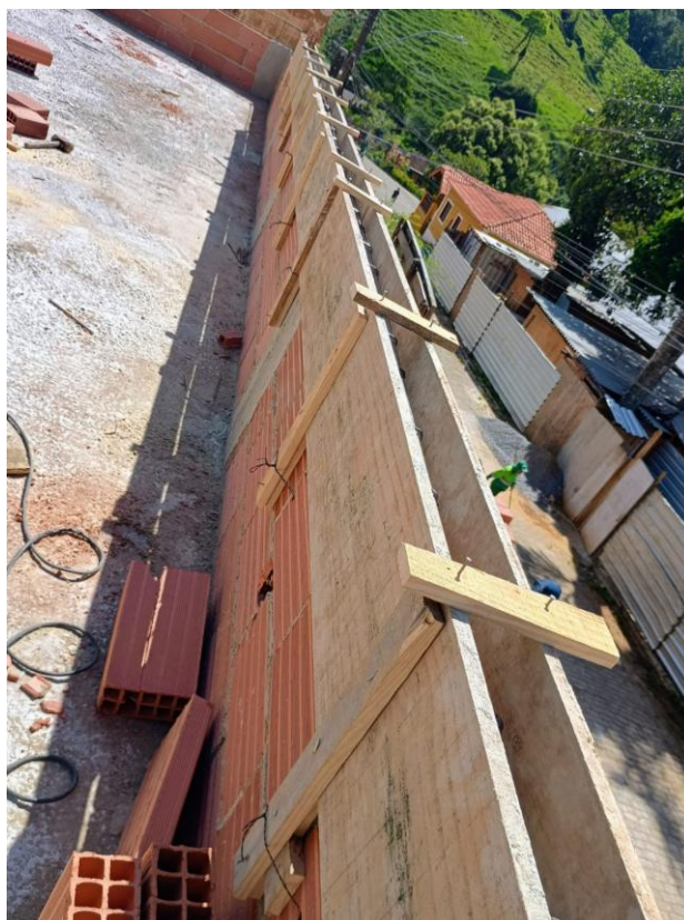
Figura 07: platibanda
