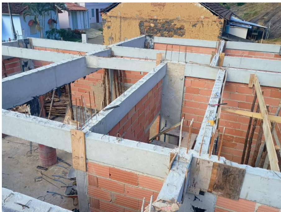
Foto 01: Vigas de cobertura
