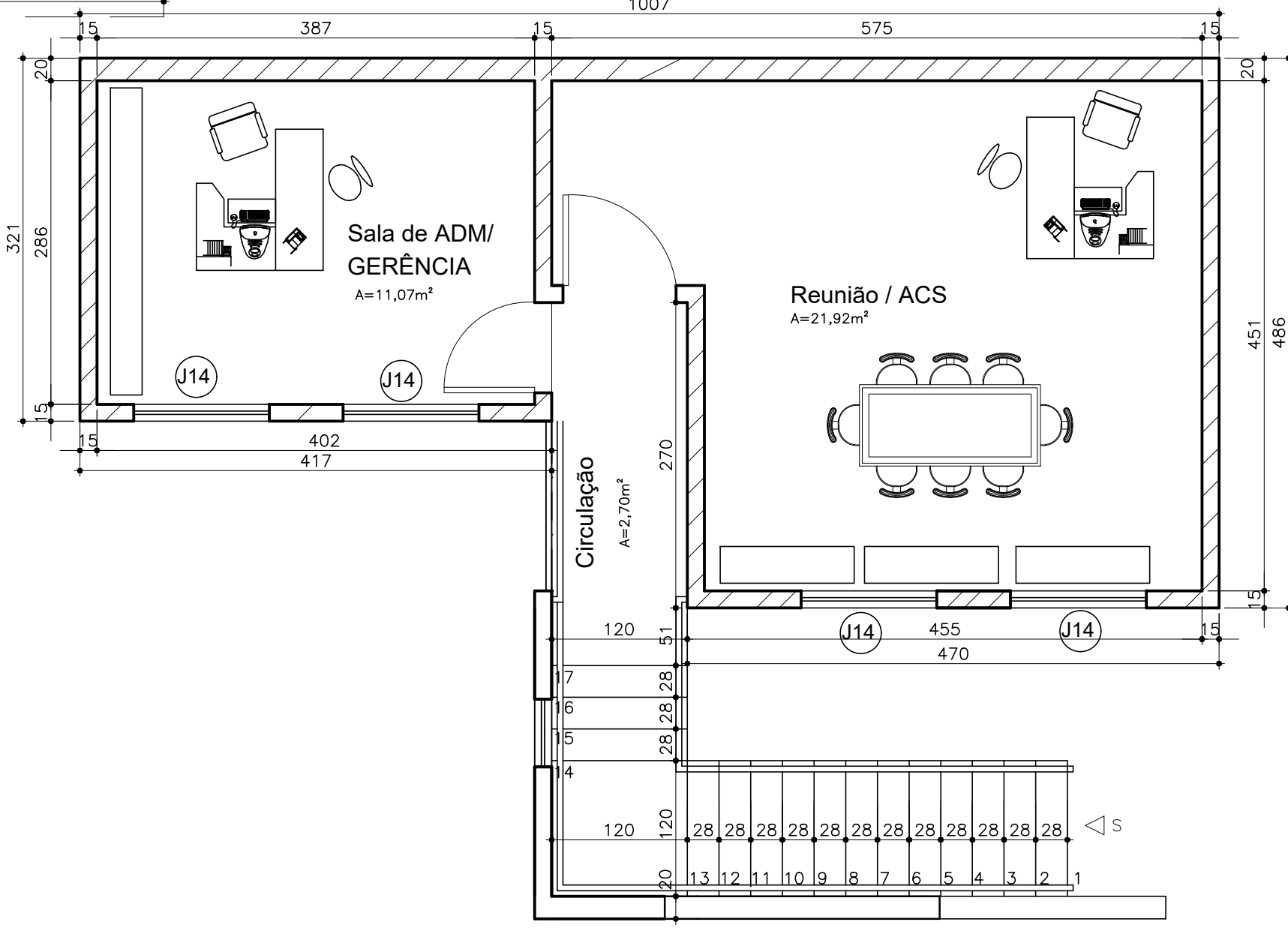
PLANTA 1º PAVIMENTO A= 41,33 m² ESCALA 1/50
