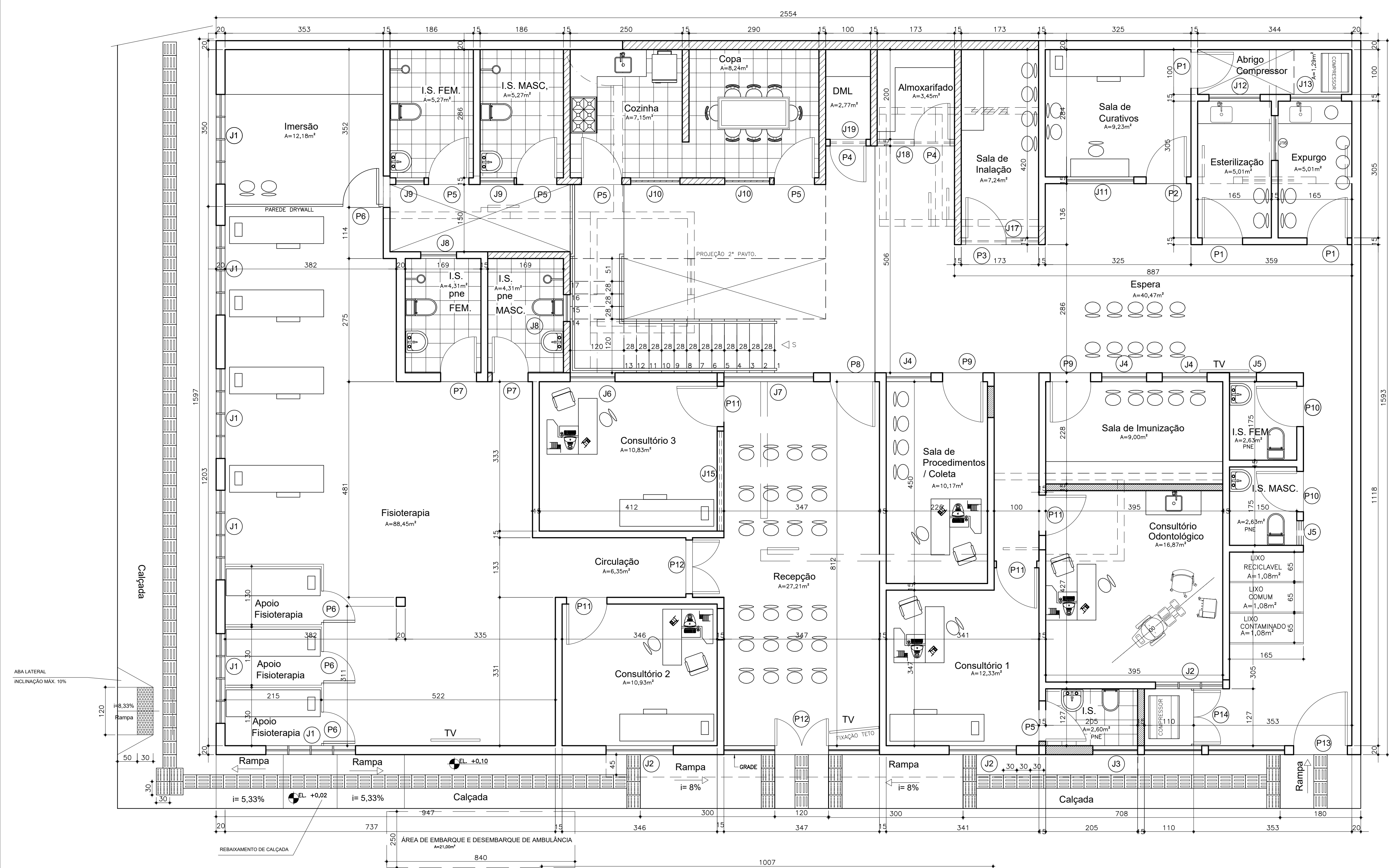
PLANTA TÉRREO A= 391,19m² ESCALA 1/50
