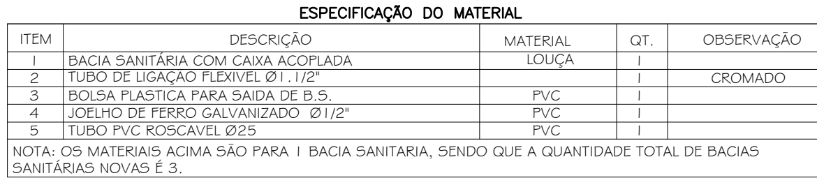
DETALHE DO VASO COM CAIXA ACOPLADA SEM ESCALA
