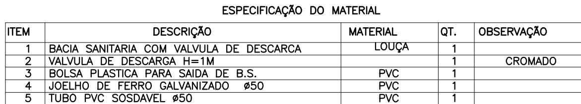
DETALHE DO VASO COM VALVULA DE DESCARGA SEM ESCALA
