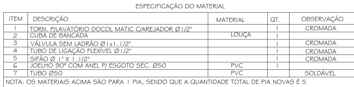
DETALHE DA PIA SEM ESCALA
