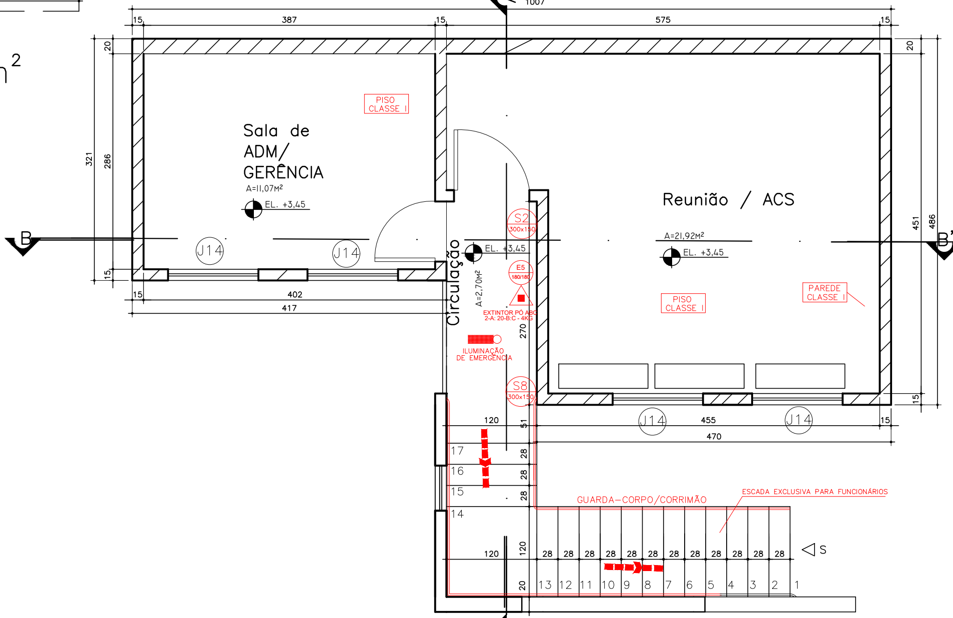
PLANTA 1º PAVIMENTO A= 41,33 m 2 ESCALA 1/50
