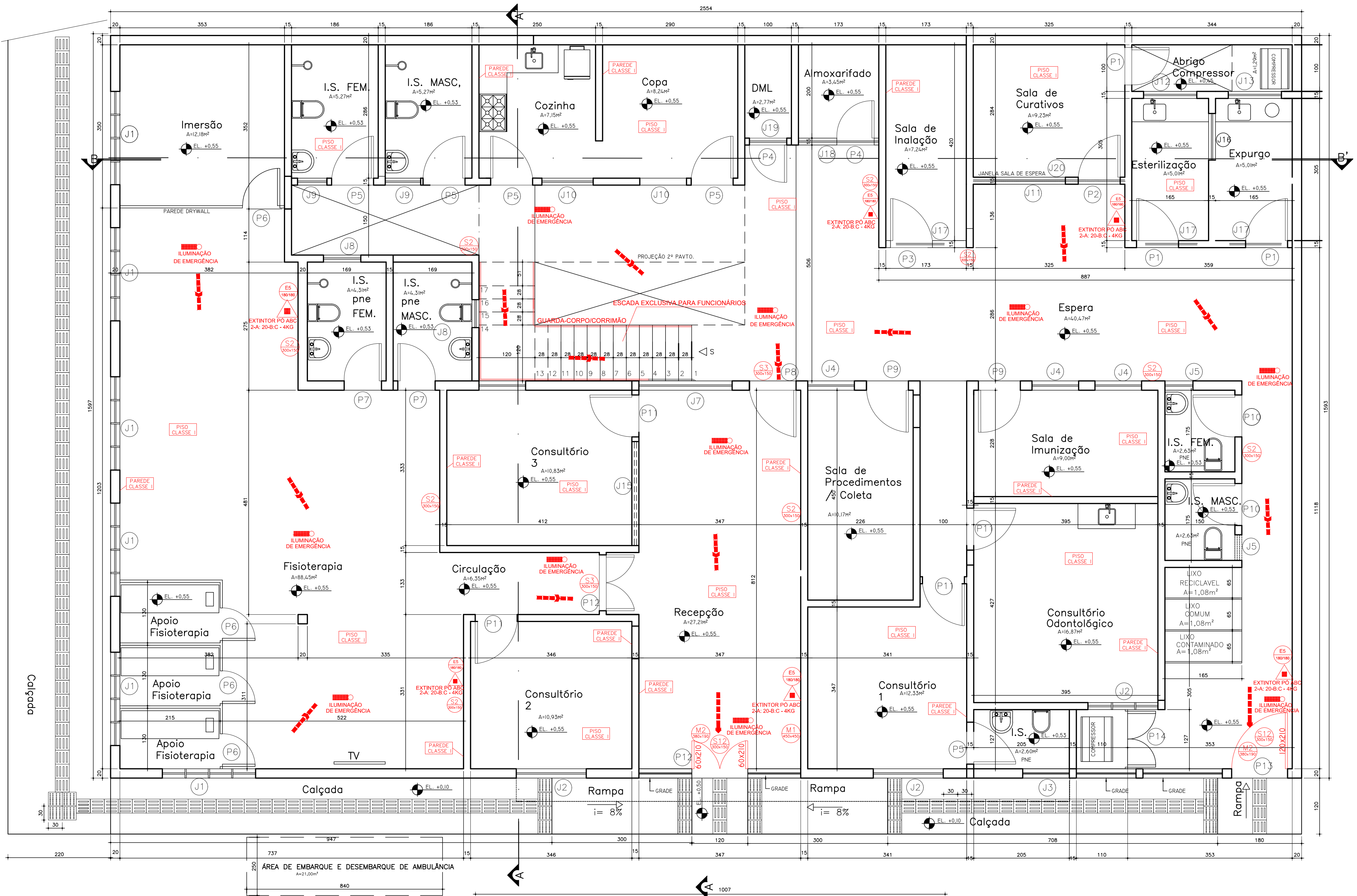
PLANTA TÉRREO A= 391,19m 2 ESCALA 1/50
