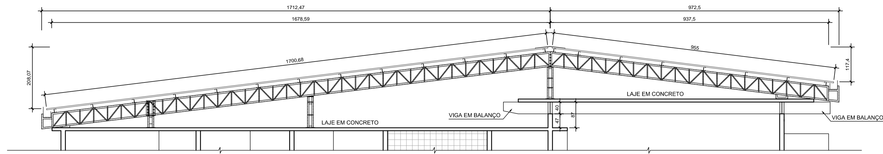
CORTE B-B' ESC. : 1/75
