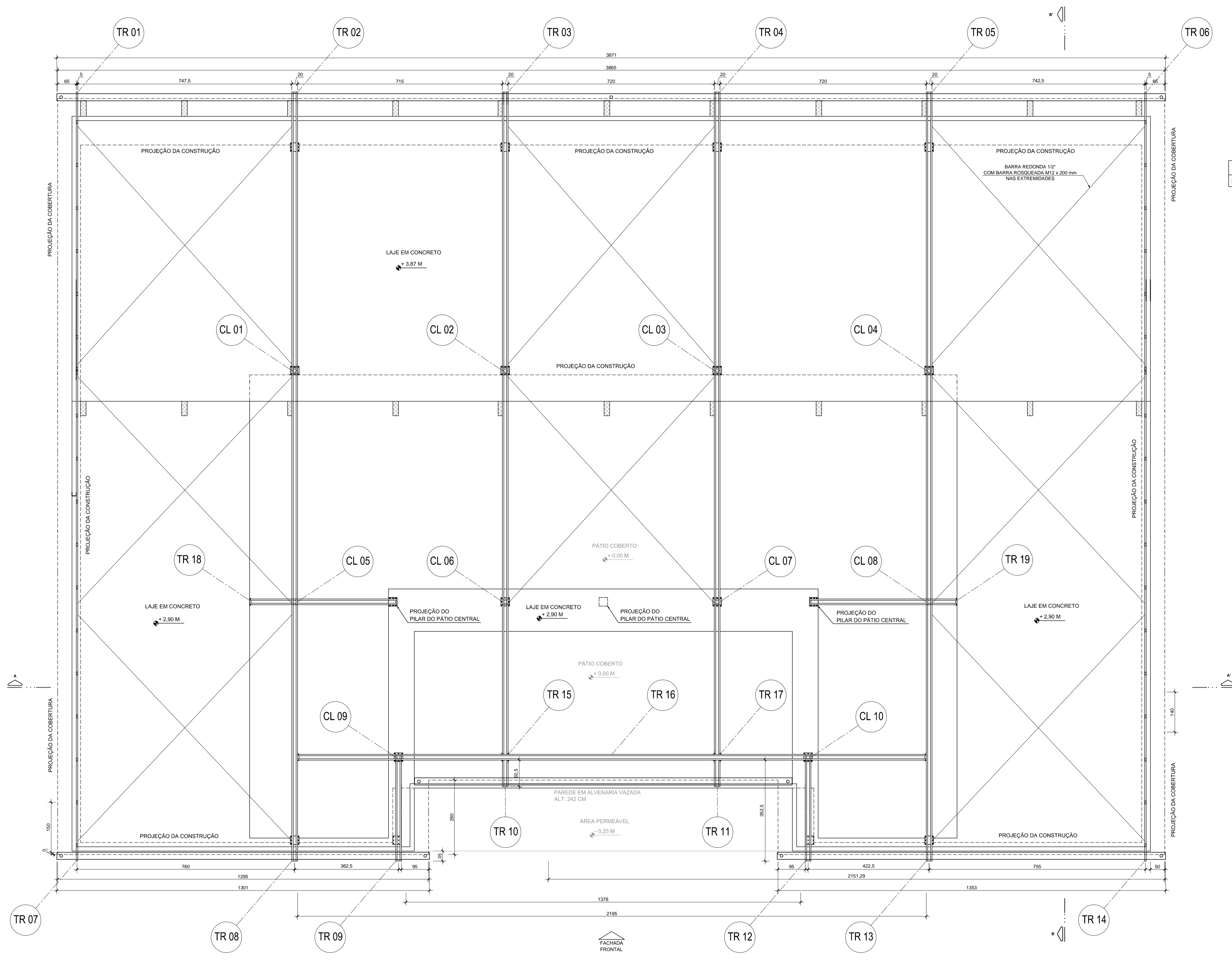
PLANTA DA ESTRUTURA METÁLICA - CONTRAVENTAMENTO ESC. : 1/75
