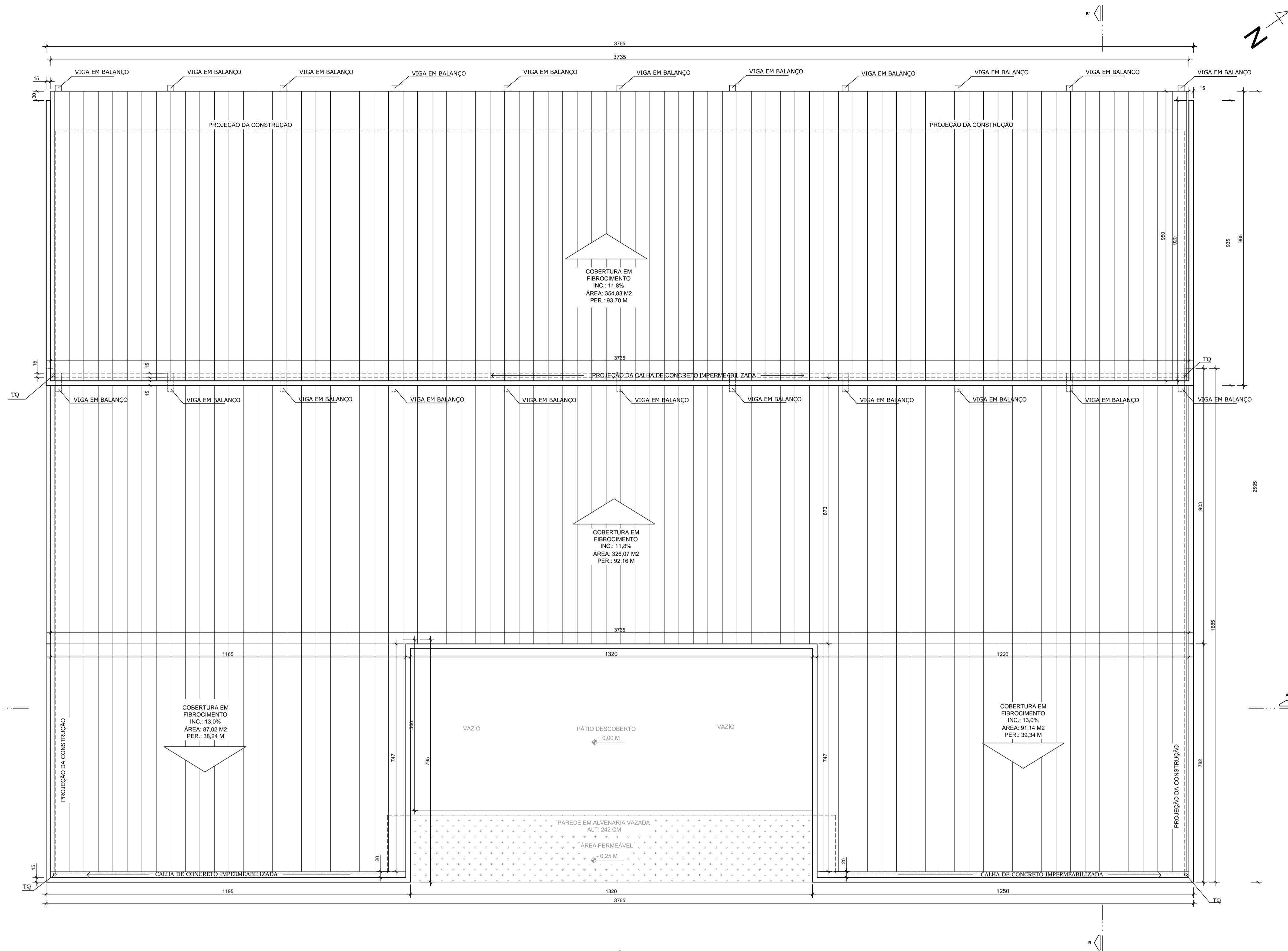
PLANTA DE COBERTURA ATUAL ESC. : 1/75
