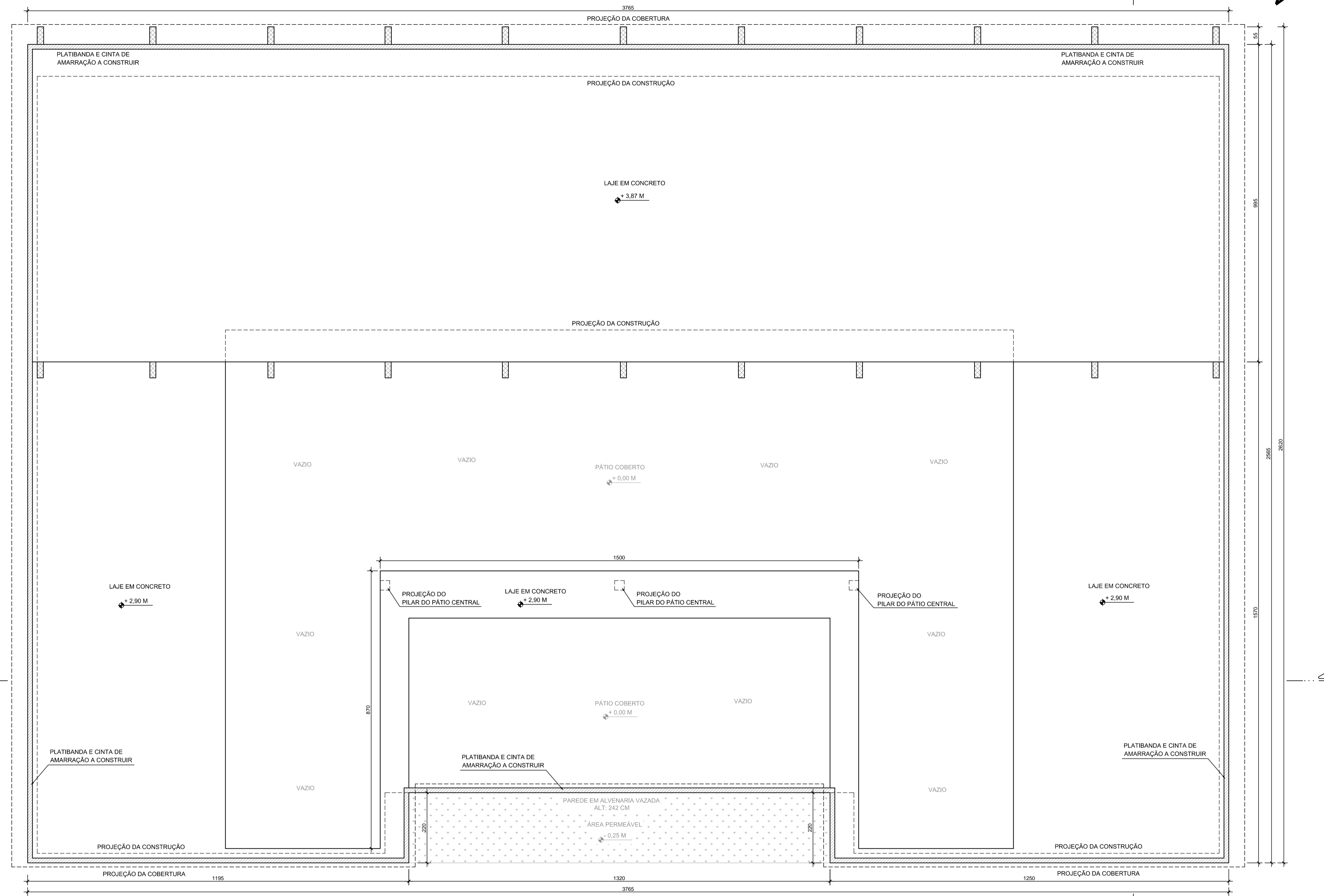
PLANTA DE CONTRUÇÃO - COBERTURA ESC. : 1/75
